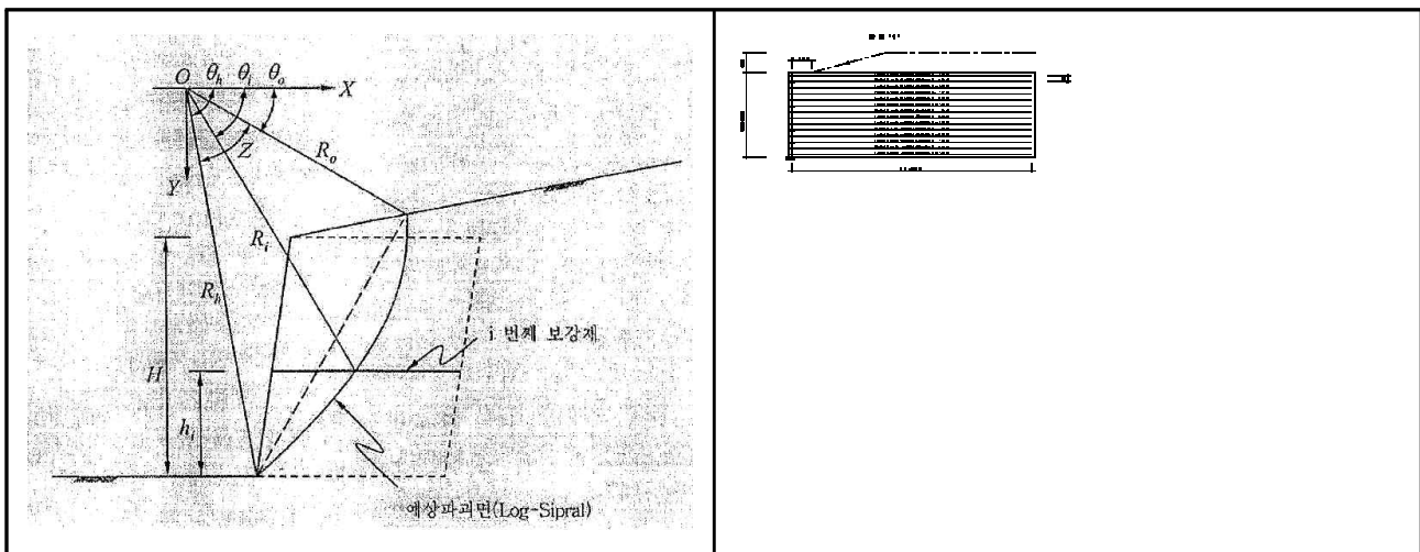
【그림 68.11】 토압작용 모식도
