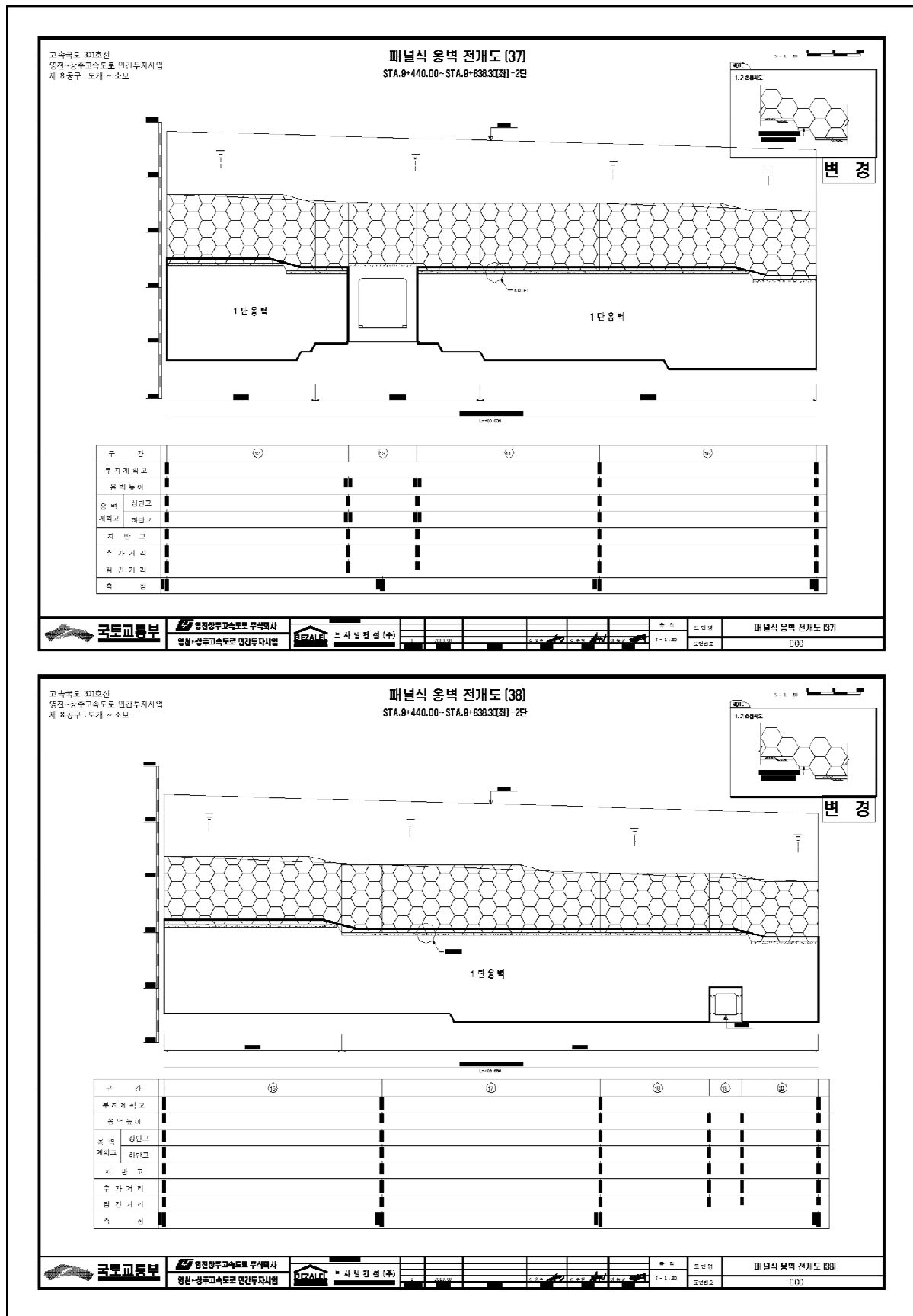
【그림 2.4】 전개도(계속)
